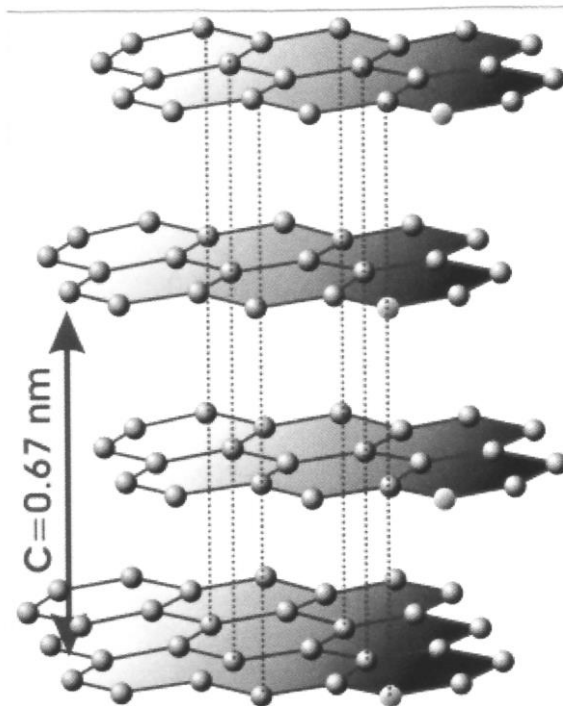
Estructura laminar del grafito (ABAB). Entre capas la interacción es débil, siendo la distancia de 3.35 \text{ \AA} , mientras que los enlaces carbono-carbono son de 1.42 \text{ \AA}
